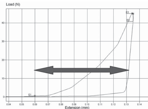
Rys. 1. Zależność siły wciskającej od przemieszczenia węgelnika. Strzałki pokazują zakres rejestracji sygnału emisji akustycznej
