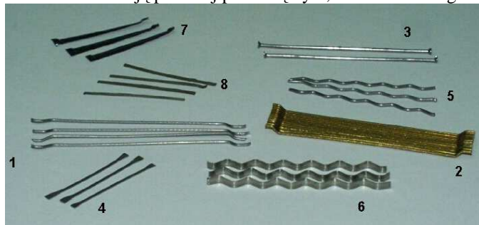
Rys.1 Przykłady kształtu włókien stalowych przeznaczonych do betonu (proste gładkie, z haczykowatymi odgięciami na obu końcach, także klejone w pasma, z zakotwieniami uformowanymi na końcach, o kształcie wiósełkowym, faliste)
