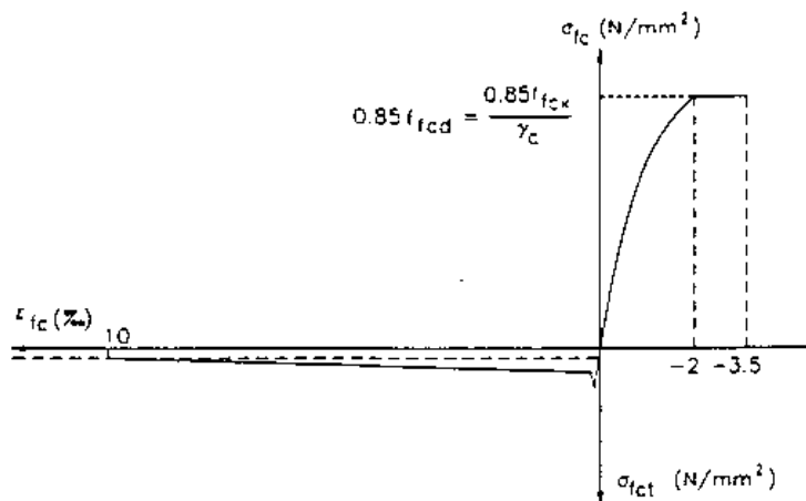
Rys. 22. Zależność konstytutywna fibrobetonu: naprężenie \sigma w funkcji odkształcenia \epsilon [11]
